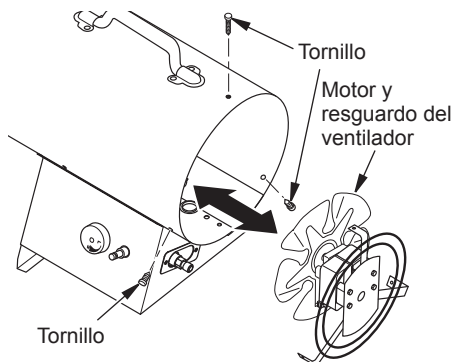
Figura 9 - Desmontaje/remplazar del motor y el resguardo del ventilador del calentador
