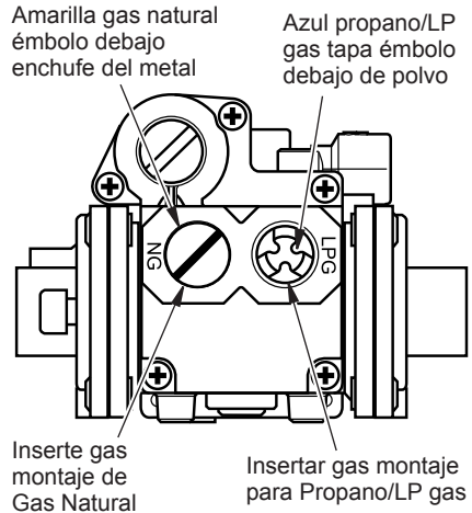
Figura 15 - Regulador de Gas
