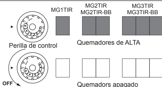
Figura 23 - Patrón del quemador
