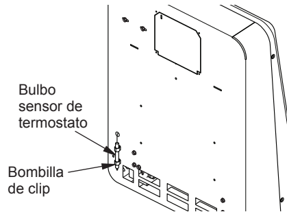
Figura 5 - Mover bulbo sensor de termostato
