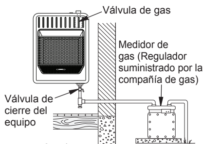
Figura 20 - Suministro de gas natural
