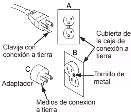
Figura 24 - Toma de corriente eléctrica con conexión a tierra
