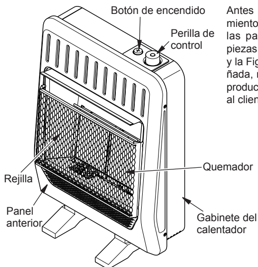
Figura 1 - Calentador de gas sin ventilación MG2TIR se muestra con la base opcional
