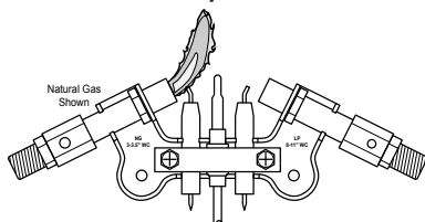
Figura 26 - Patrón incorrecto de la llama del piloto
