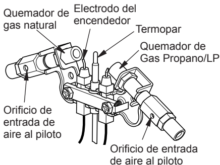
Figura 22 - Conjunto de piloto
