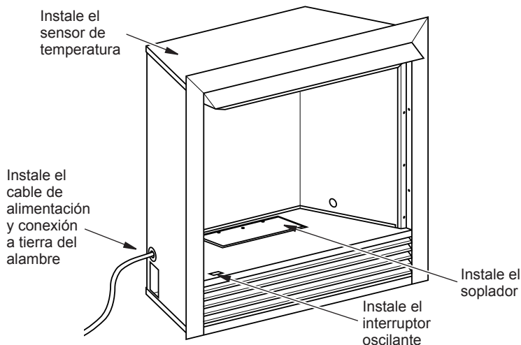
Blower Asamblea Posición de instalación para PC32VFC y PC36VFC Solo Series
