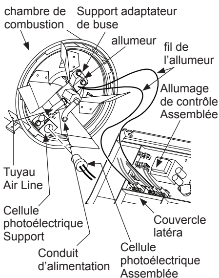
Figure 14 - débrancher les fils de l'allumeur Assemblée de contrôle d'allumage
