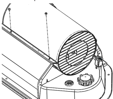
Figura 7 - Desmontaje de la cubierta superior
