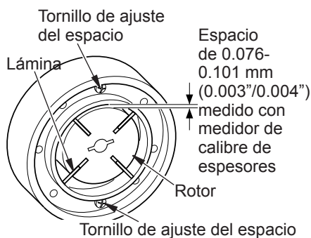
Figura 21 - Ubicaciones del tornillo de ajuste del espacio
