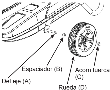
Figura 2 - Montaje de la rueda, los modelos 160, 175 y 220
