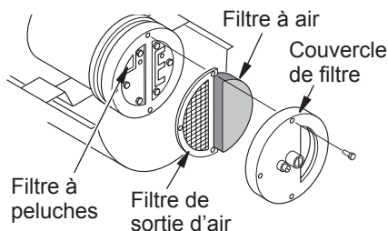
Figure 10 - Filtres de sortie d'air, d'admission d'air, et les peluches
