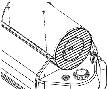
Figure 7 - Enlèvement coque supérieure
