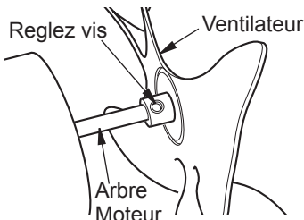
Figure 8 - Fan, arbre du moteur, et l'emplacement Vis
