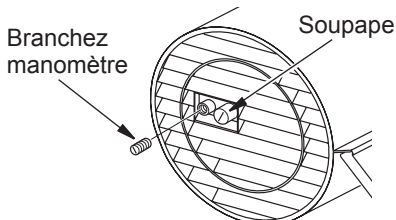
Figure 11 - retrait de la prise manomètre
