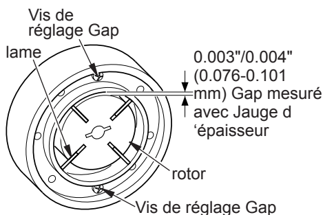
Figure 21 - Emplacements Gap Vis de réglage
