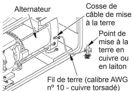
Figure 6 - Méthode typique de mise à la terre du générateur (la construction du générateur pourrait être différente de l'illustration)
