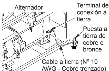
Figura 15 - Método de conexión a tierra habitual del generador (la estructura del generador puede diferir de la imagen que se muestra)
