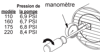
Figure 12 - Réglage de la pression de la pompe
