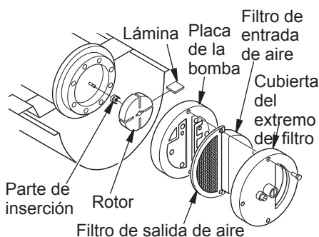
Figura 20 - Ubicación del rotor
