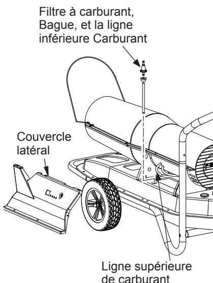
Figure 13 - Retrait du filtre Carburant
