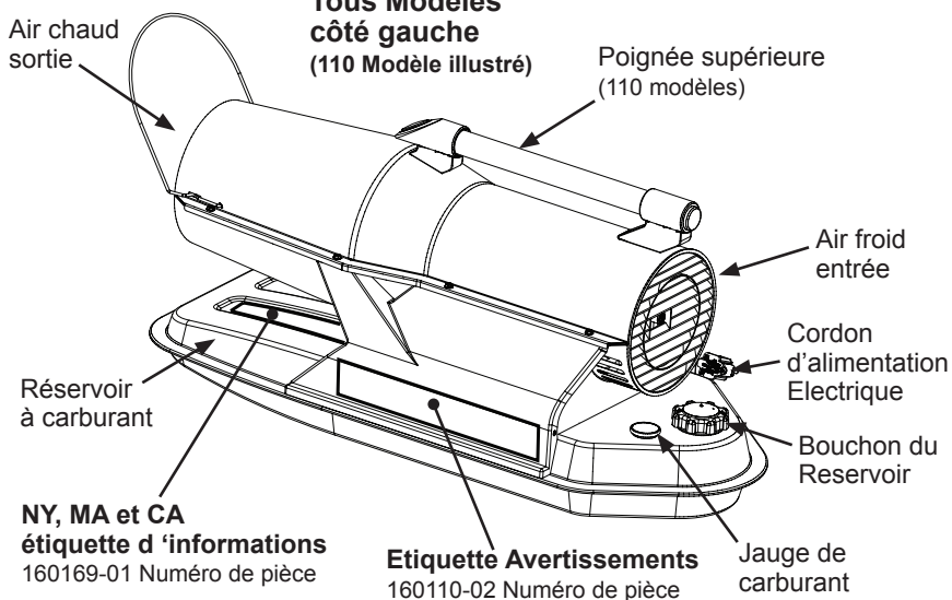
Figure 4 - Identification du produit et Emplacement des étiquettes
