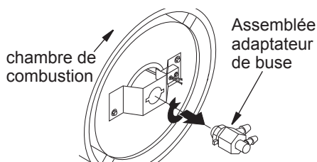
Figure 17 - Retrait de Assemblée adaptateur de buse
