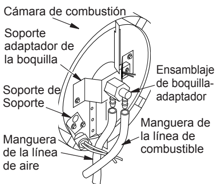
Figura 16 - Desmontaje de las mangueras de las líneas de aire y combustible
