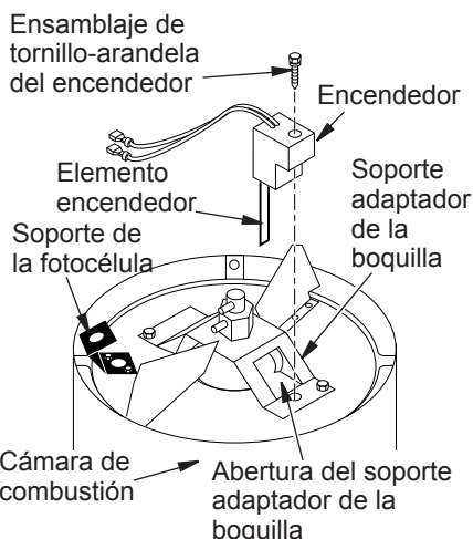
Figura 15 - Reemplazo del encendedor
