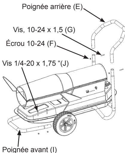
Figure 3 - Assemblée Poignée, les modèles 160, 175 et 220
