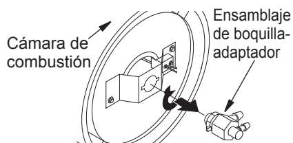
Figura 17 - Desmontaje del ensamblaje de la boquilla-adaptador
