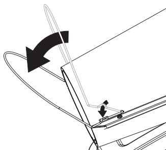
Figura 1 - Guarda de alambre trasladado a posición de bloqueo
