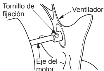
Figura 8 - Ubicación del ventilador, del eje del motor y del tornillo de fijación
