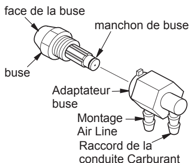
Figure 18 - La buse et adaptateur de buse
