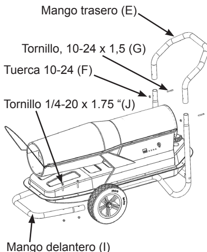
Figura 3 - Manija, los modelos 160, 175 y 220
