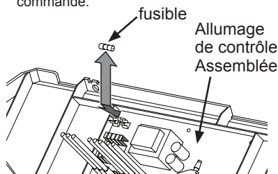
Figure 19 - Remplacement du fusible
