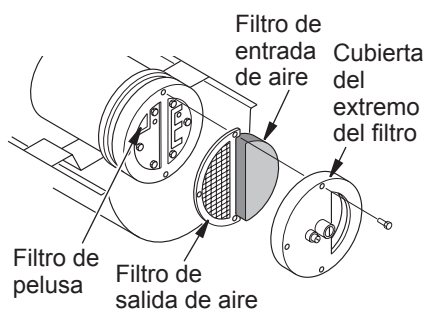
Figura 10 - Filtros de salida de aire, entrada de aire y de pelusa
