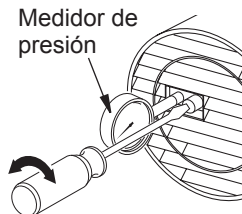
Figura 12 - Ajuste de la presión de la bomba
