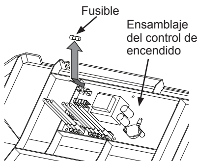
Figura 19 - Reemplazo del fusible
