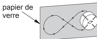
Figure 22 - Ponçage du rotor
