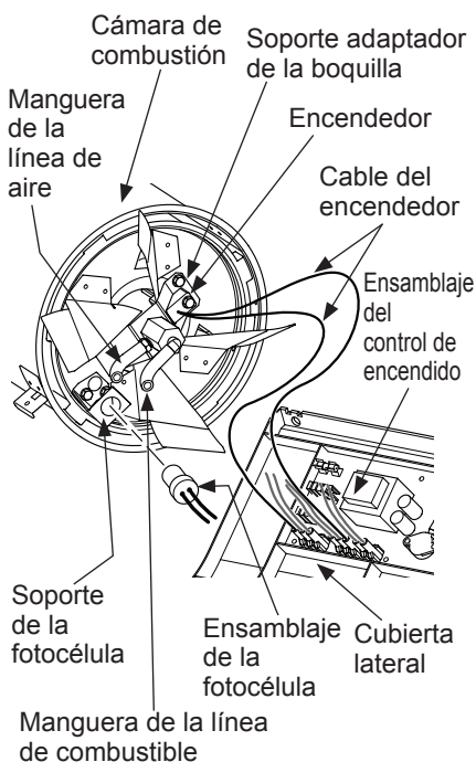
Figura 14 - Desconexión de los cables del encendedor del ensamblaje del control de encendido
