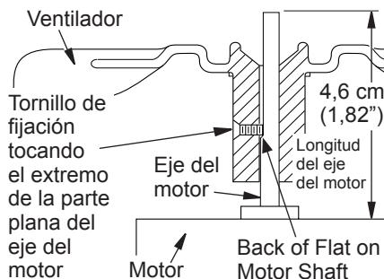
Figura 9 - Vista transversal del ventilador
