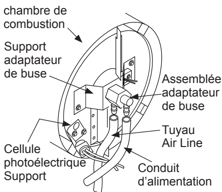
Figure 16 - Retrait de l'air et les tuyaux souples de Carburant
