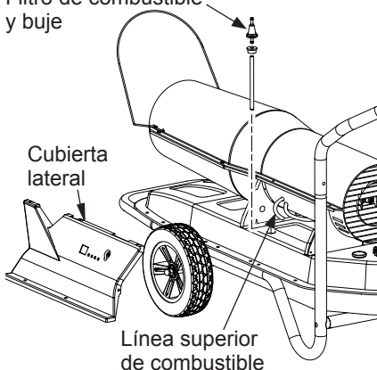
Figura 13 - Desmontaje del filtro de combustible
