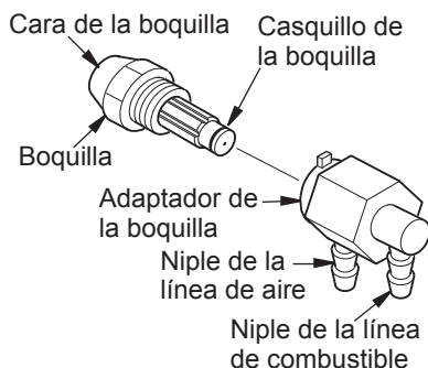
Figura 18 - Boquilla y adaptador de la boquilla
