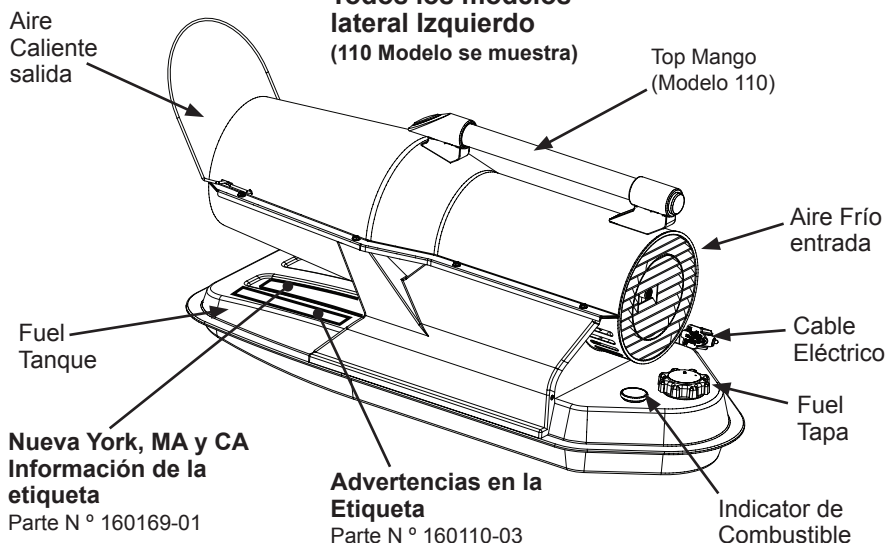
Figura 4 - Identificación del Producto y Ubicación de las etiquetas
